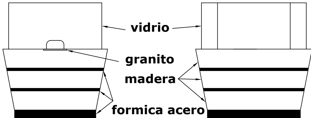
FACHADAS LATERALES
