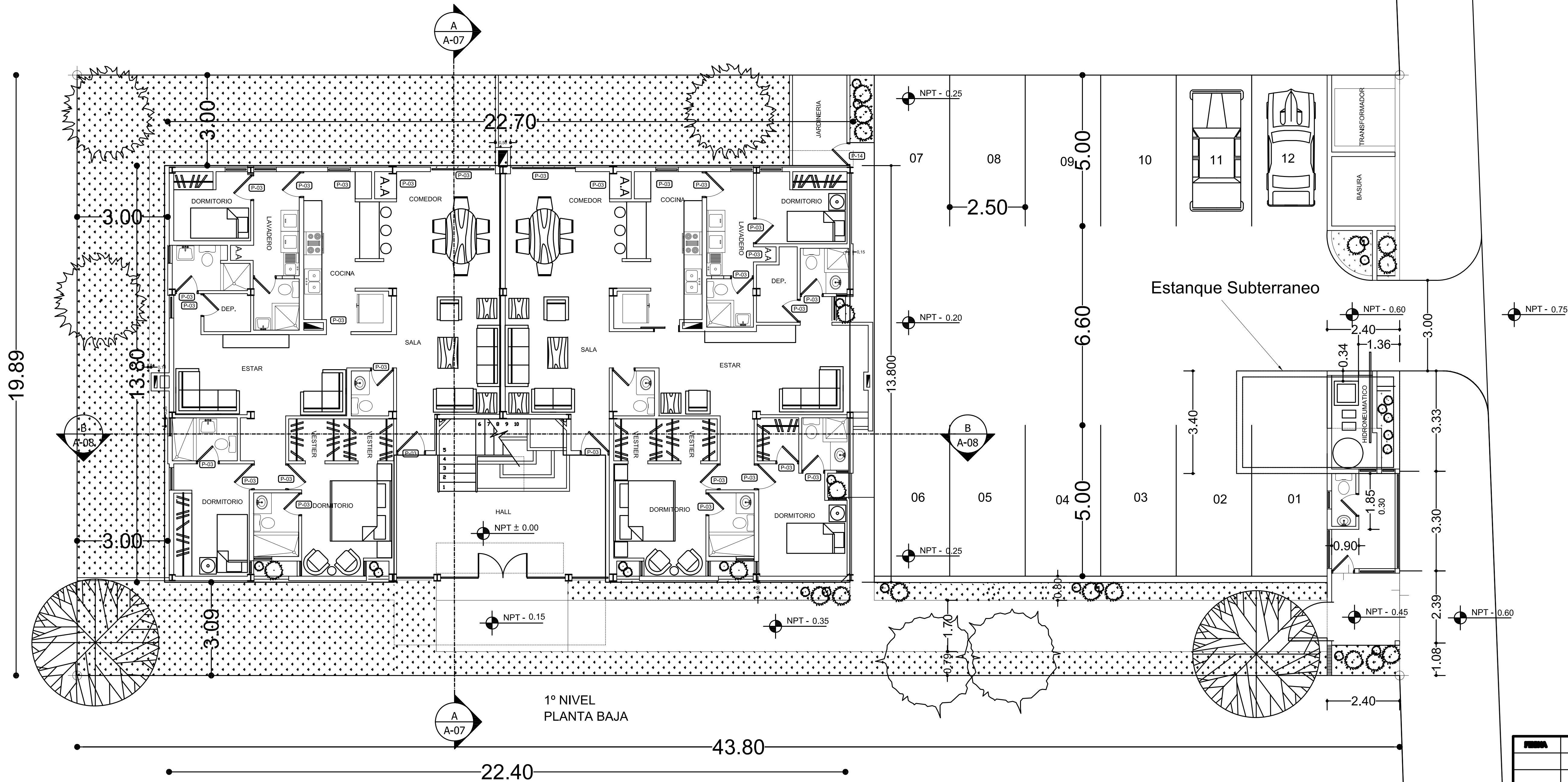
PLANTA GENERAL
