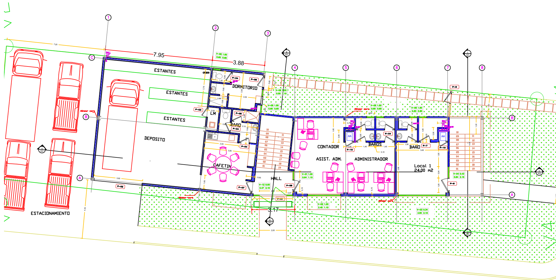
Planta Baja
