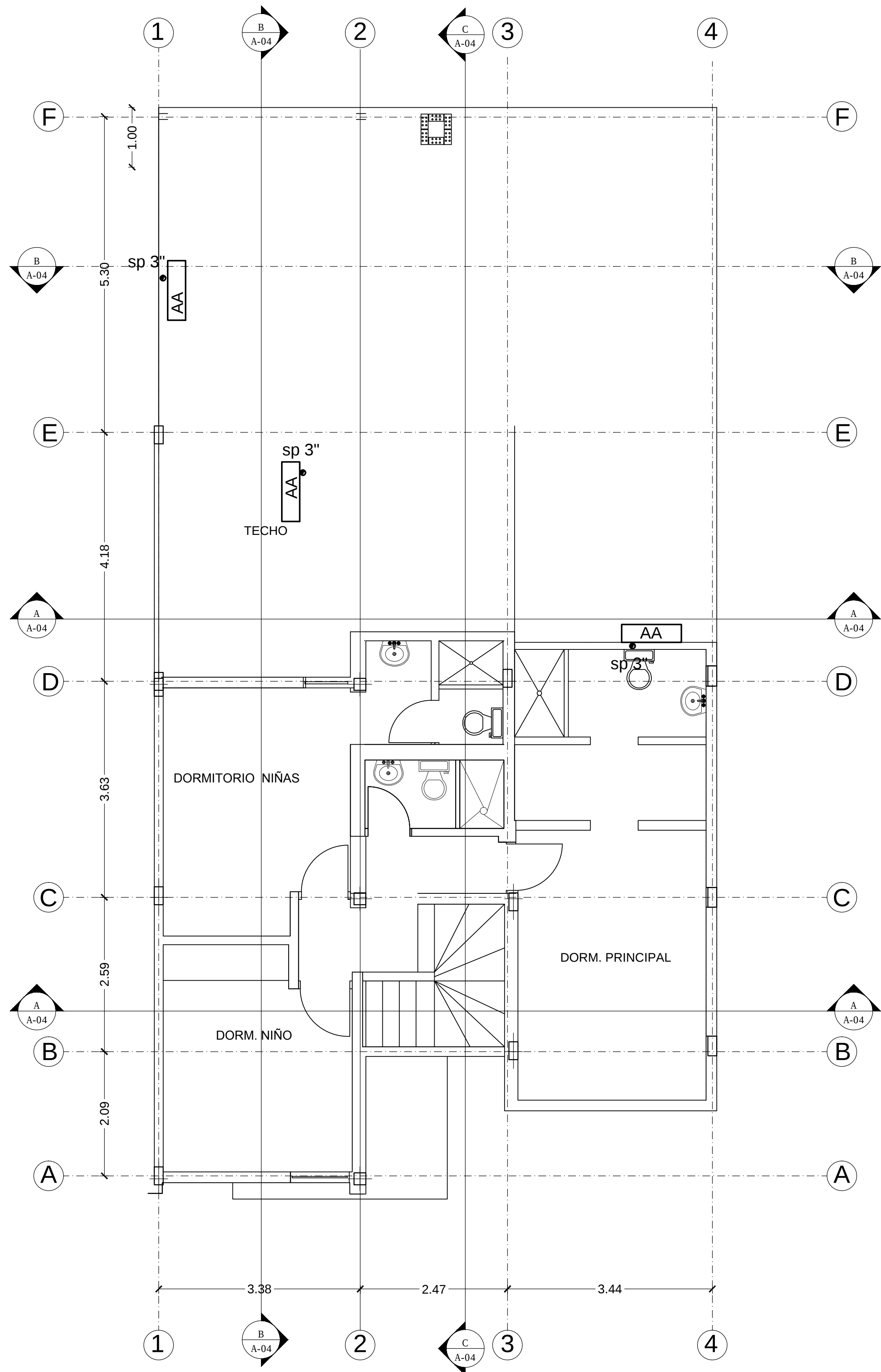
PLANTA ALTA ACTUAL
