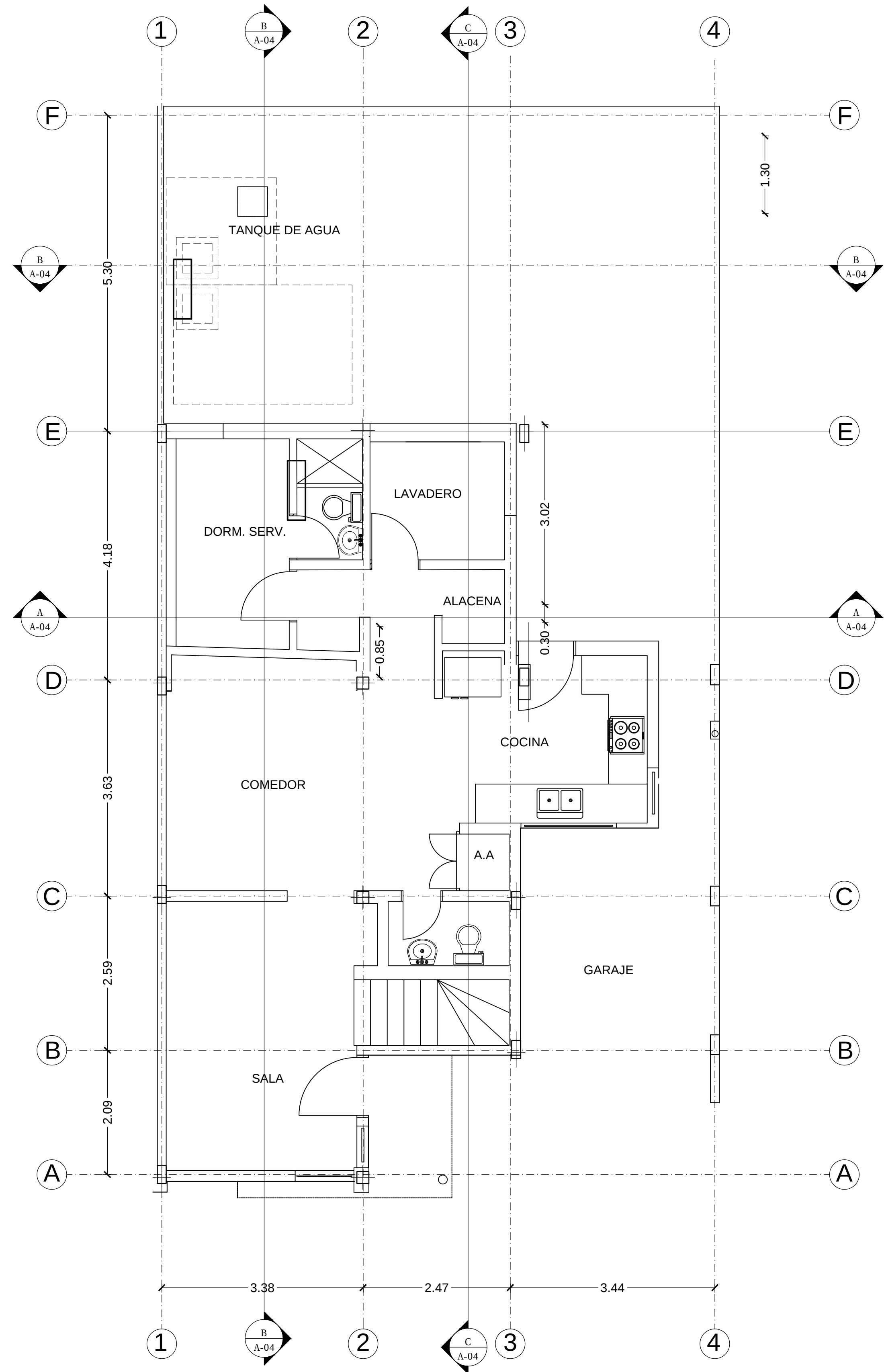
PLANTA BAJA ACTUAL
