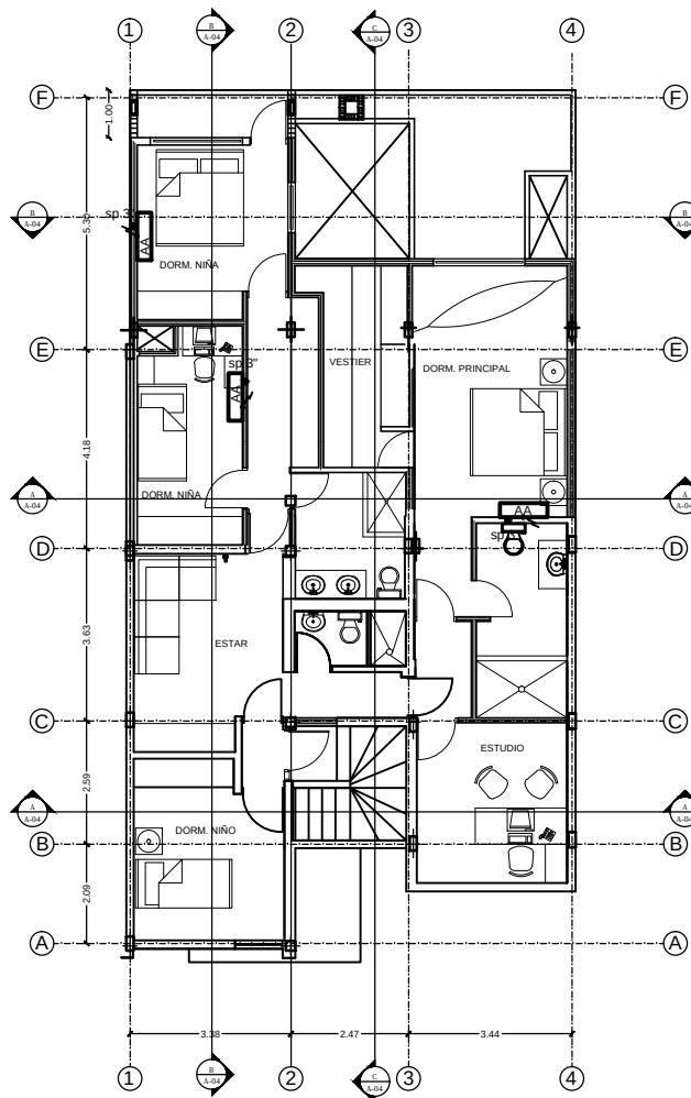
PLANTA ALTA PROPUESTA
