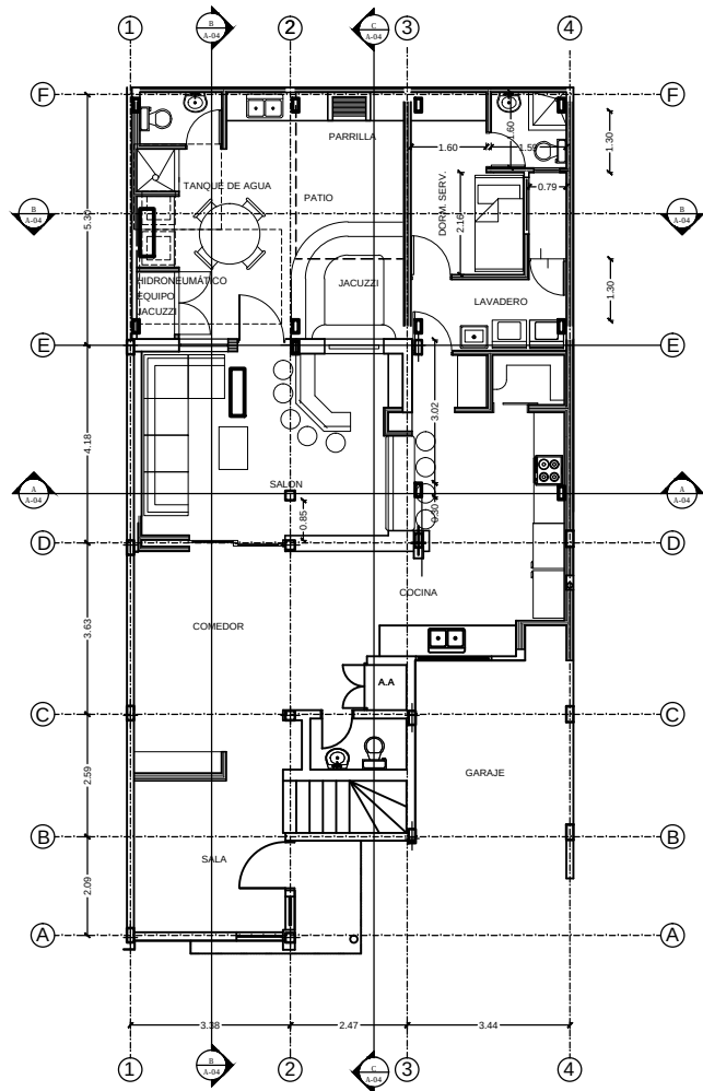
PLANTA BAJA PROPUESTA
