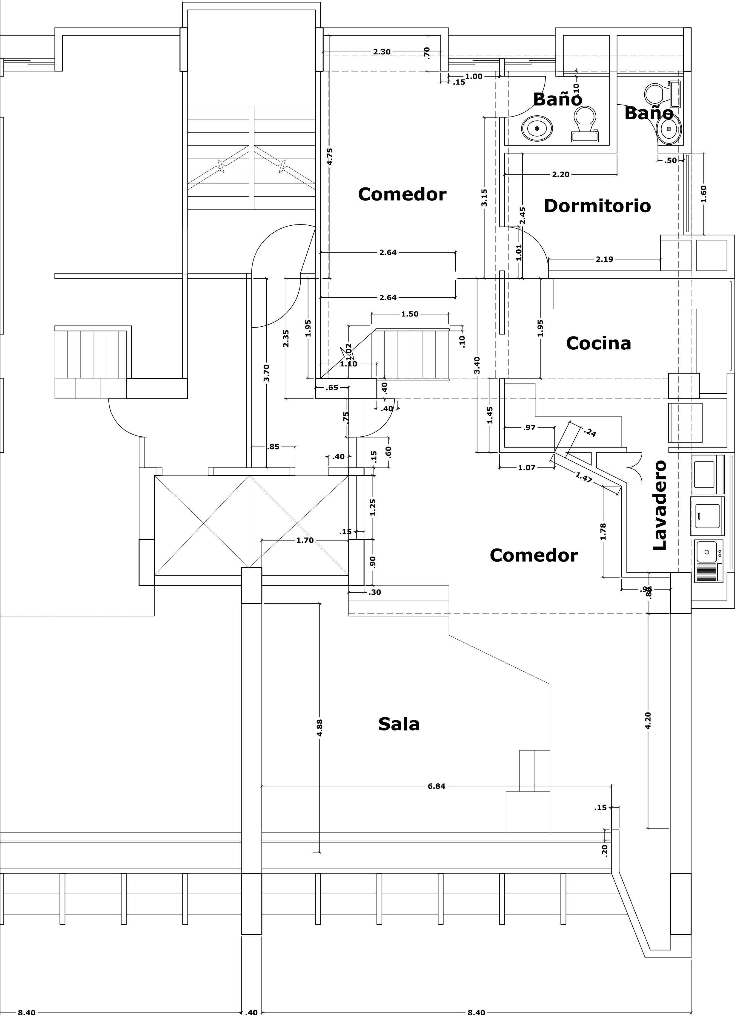
PLANTA BAJA ACTUAL
