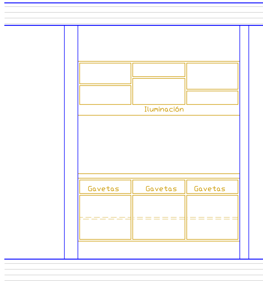
CORTE C-2
