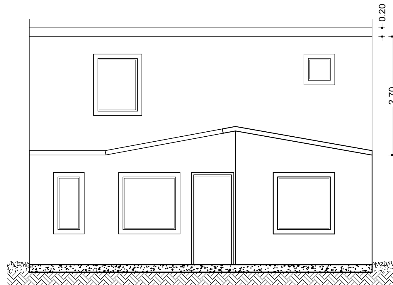
FACHADA PROPUESTA
